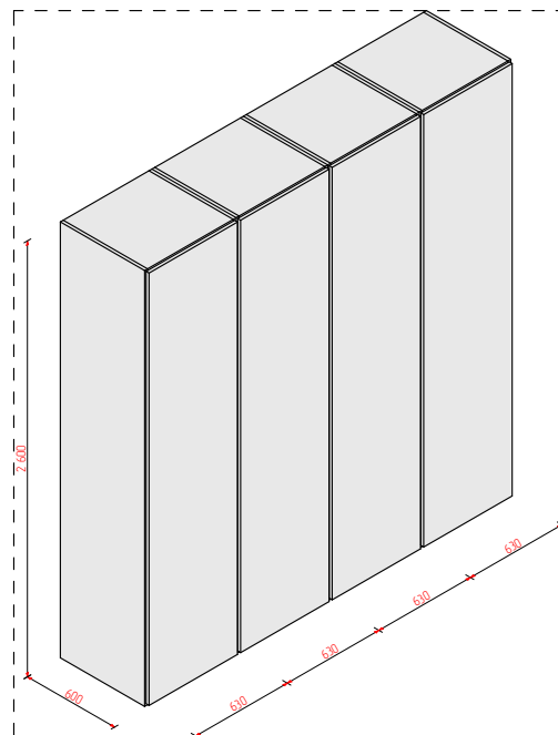
7 Деталь q 1:50
