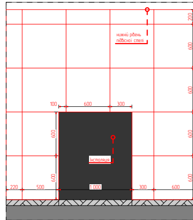
03 Розгортка 1:50
