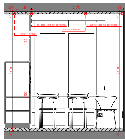
9 Перетин (1) 1:50
