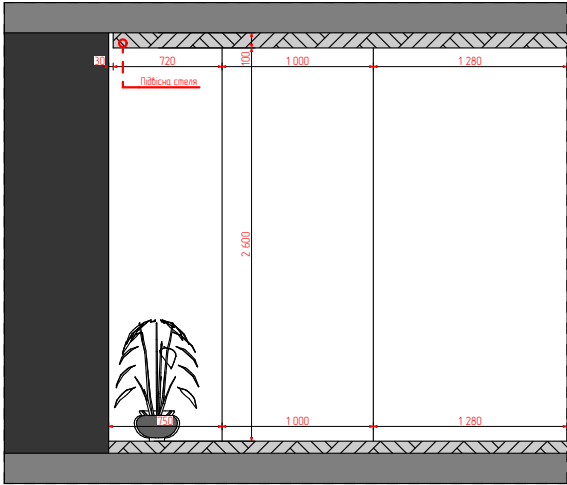
2 Перетин (1) 1:50
