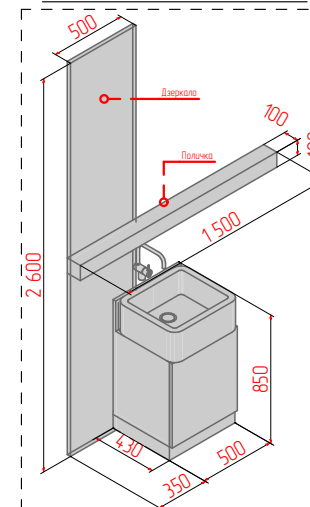
11 Деталь 1:50
