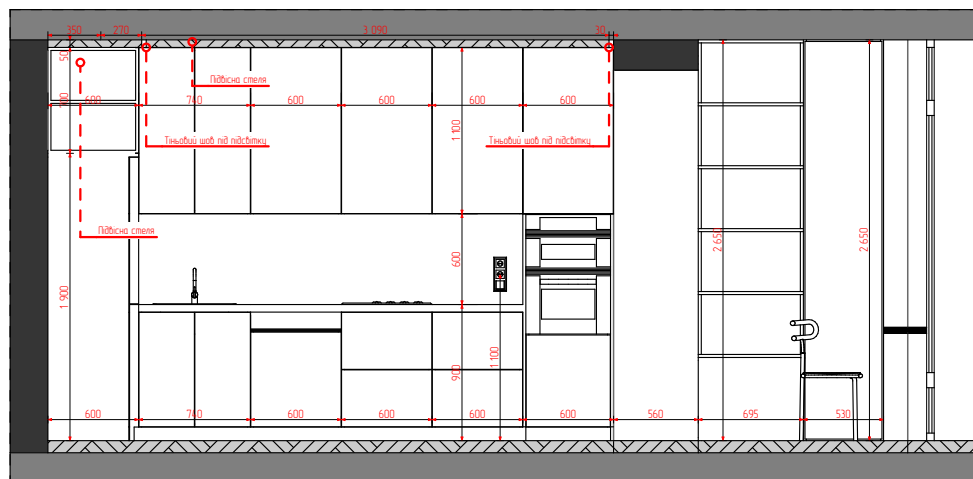
8 Перетин (1) 1:50
