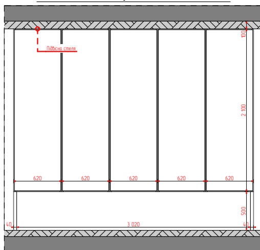
13 Перетин 1:50
