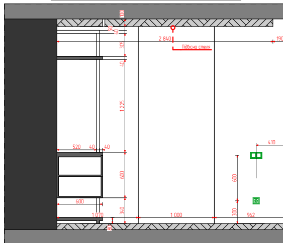
18 Перетин 1:50
