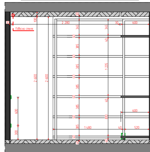
19 Перетин 1:50
