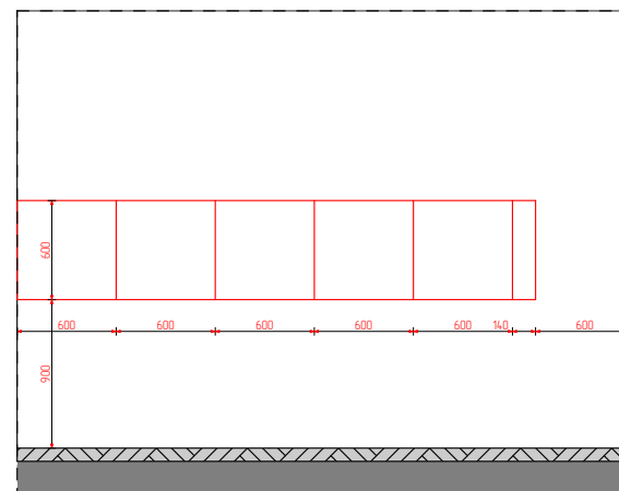
010 Розгортка 1:50
