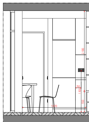
12 Перетин (1) 1:50
