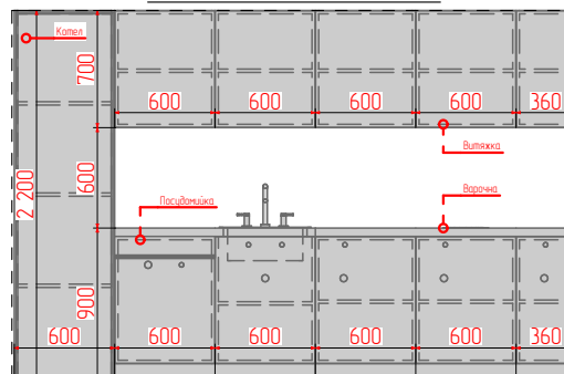
3 Деталь w 1:50
