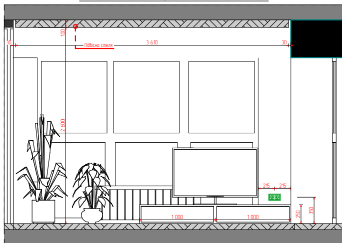
23 Перетин 1:50
