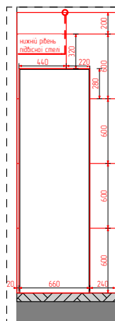
08 Розгортка 1:50
