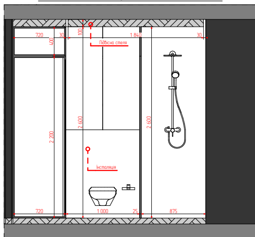
9 Перетин 1:50
