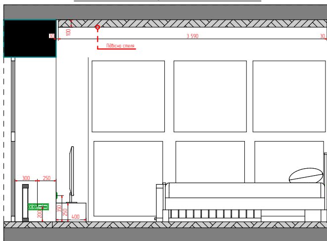
24 Перетин 1:50
