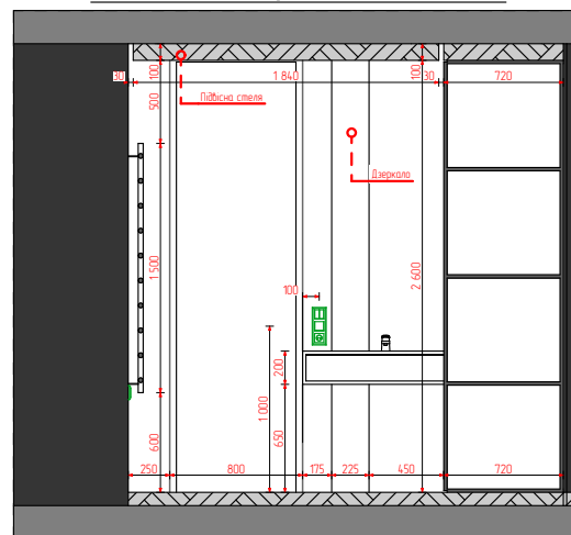
11 Перетин 1:50
