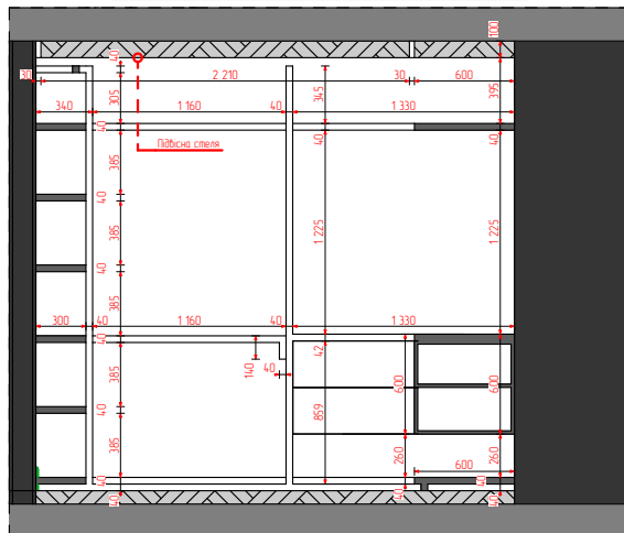
20 Перетин 1:50
