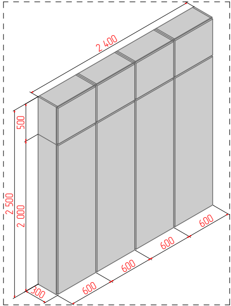
7 Деталь q 1:50
