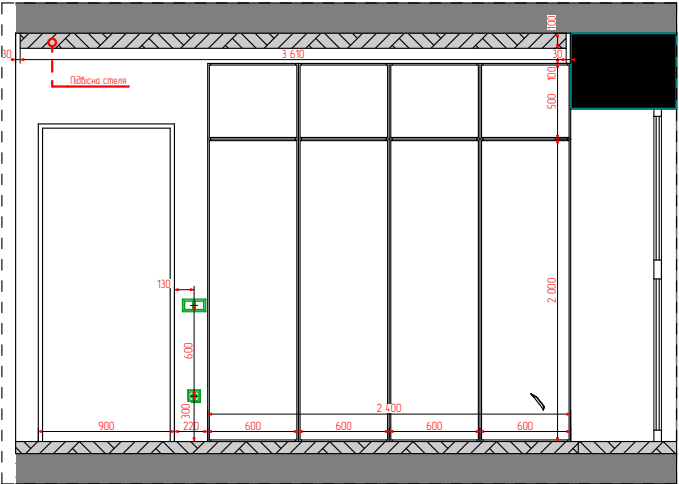
4 Перетин 1:50
