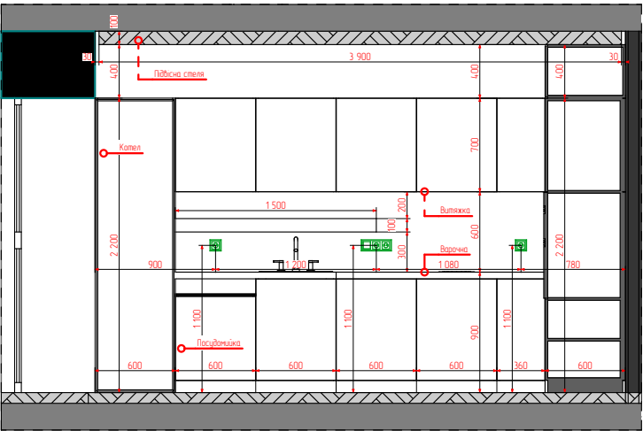
6 Перетин 1:50
