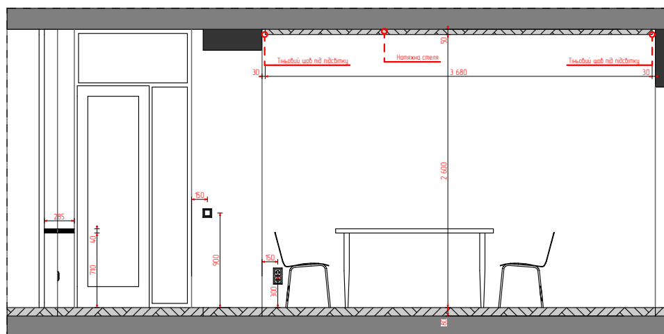
11 Перетин (1) 1:50
