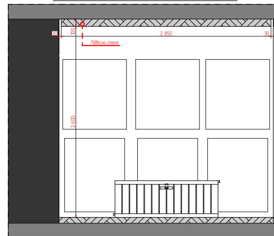
28 Перетин 1:50
