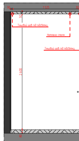
22 Перетин (1) 1:50
