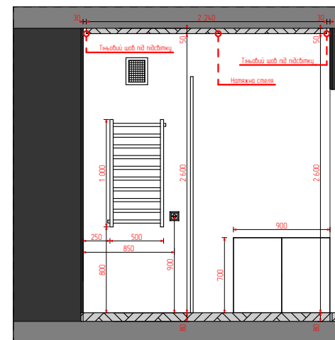
23 Перетин (1) 1:50
