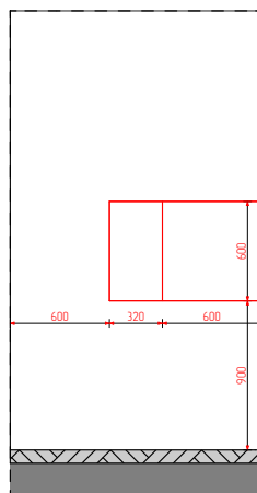
09 Розгортка 1:50
