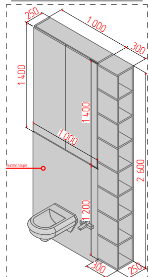
12 Деталь q 1:50
