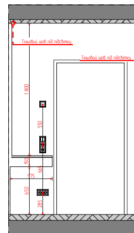
6 Перетин (1) 1:50
