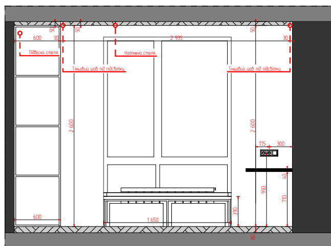
18 Перетин (1) 1:50
