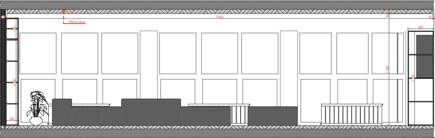
5 Перетин 1:50
