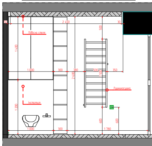
27 Перетин 1:50
