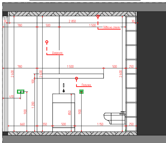
26 Перетин 1:50
