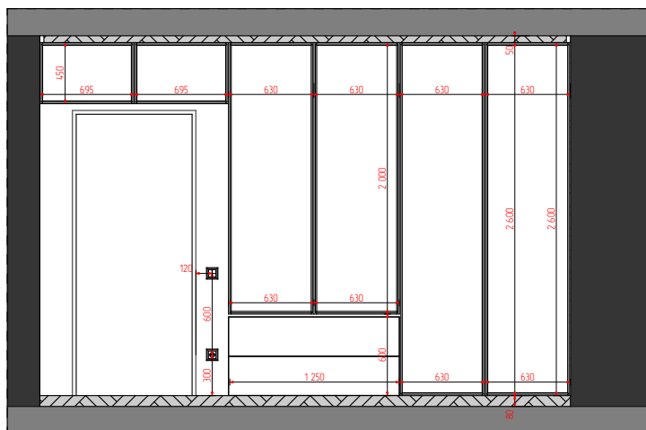
31 Перетин 1:50
