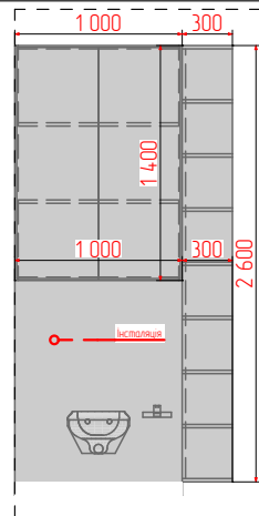
12 Деталь w 1:50
