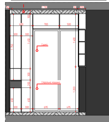
12 Перетин 1:50
