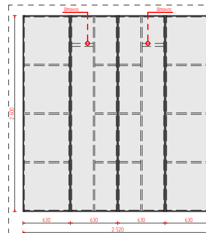
7 Деталь w 1:50
