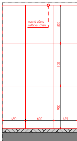
02 Розгортка (1)1:50
