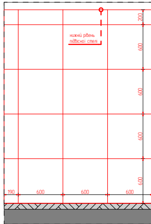
01 Розгортка 1:50
