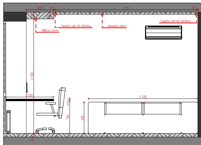
15 Перетин (1) 1:50
