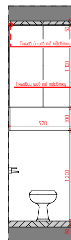
27 Перетин (1) 1:50
