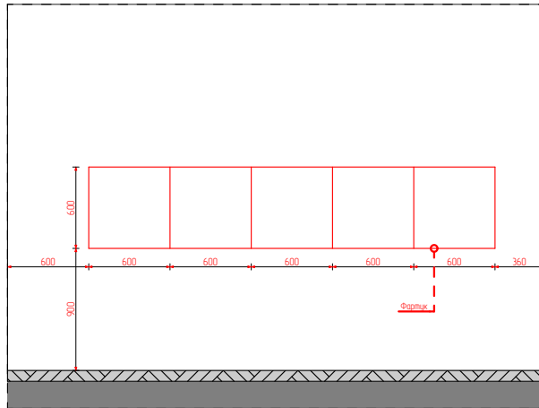
07 Розгортка 1:50
