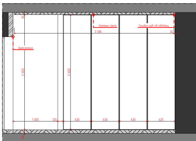
17 Перетин (1) 1:50
