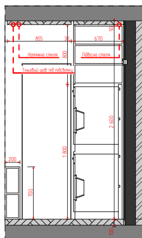
24 Перетин (1) 1:50
