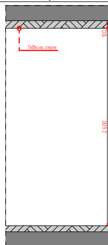
15 Перетин 1:50
