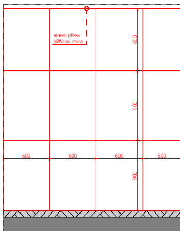
03 Розгортка (1)1:50
