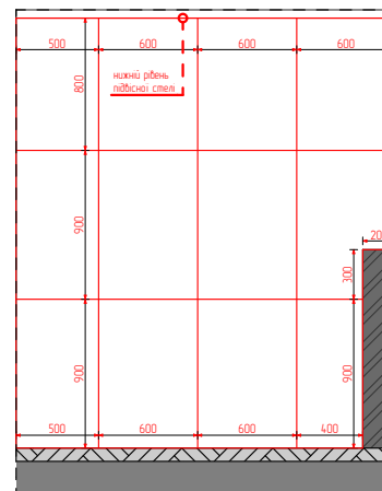
05 Розгортка (1)1:50
