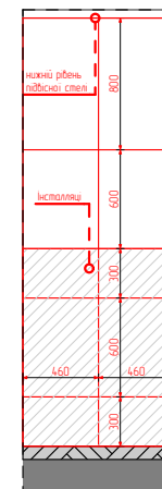
06 Розгортка (1)1:50
