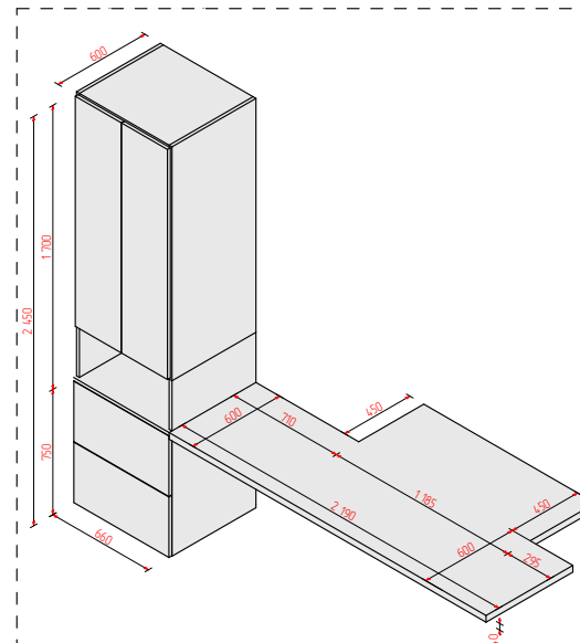
7 Деталь w 1:50
