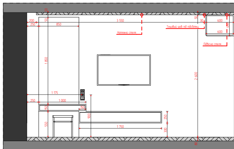
34 Перетин 1:50
