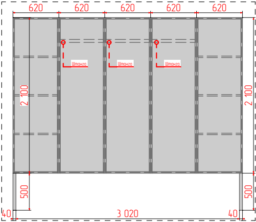
6 Деталь w 1:50
