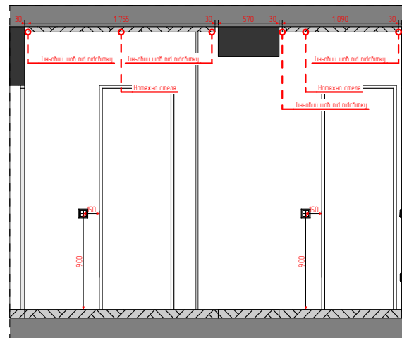
2 Перетин (3) 1:50
