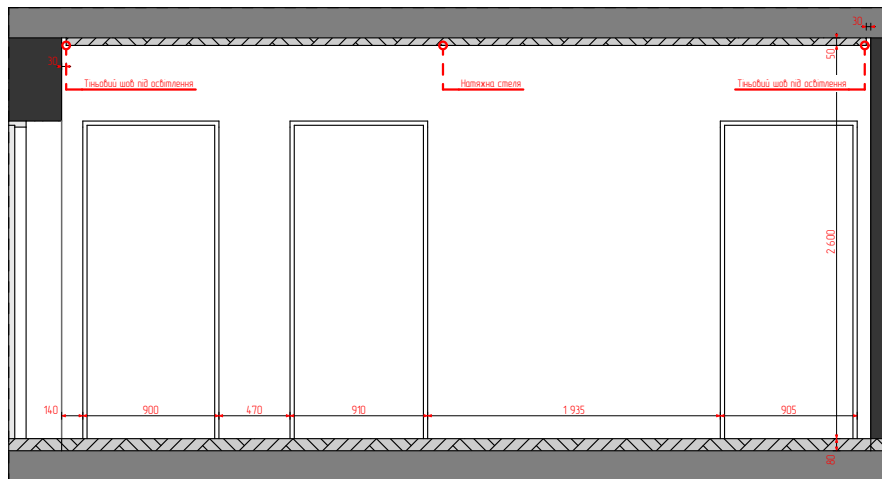
1 Перетин (1) 1:50
