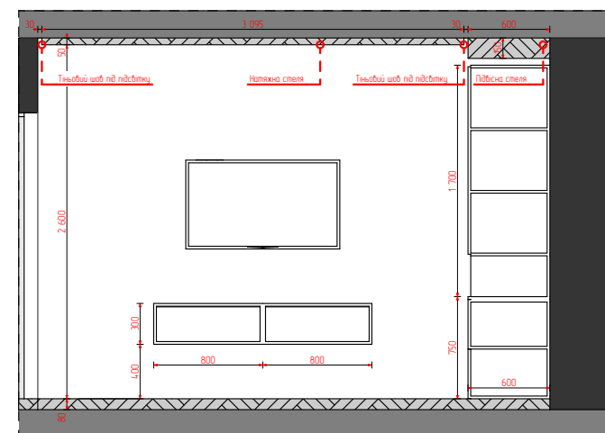
13 Перетин (1) 1:50
