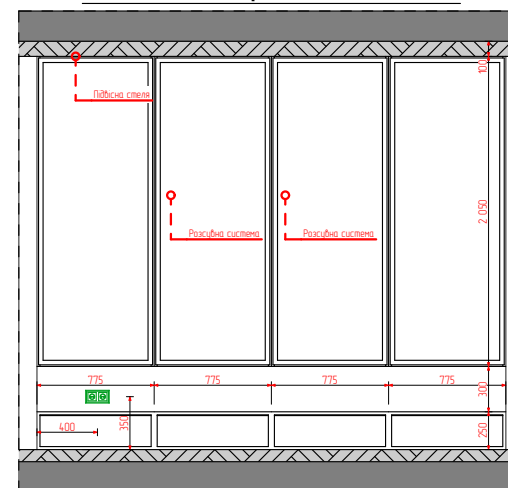
16 Перетин 1:50
