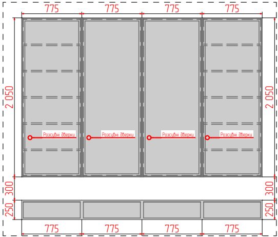
5 Деталь w 1:50
