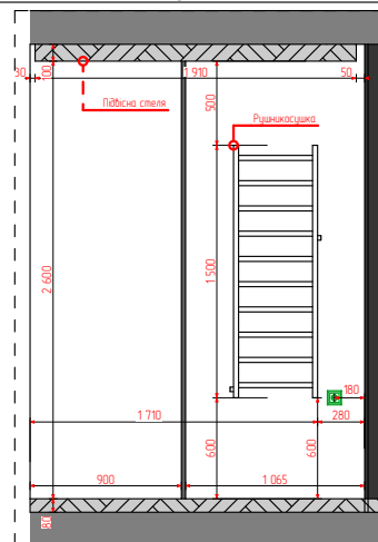
10 Перетин 1:50
