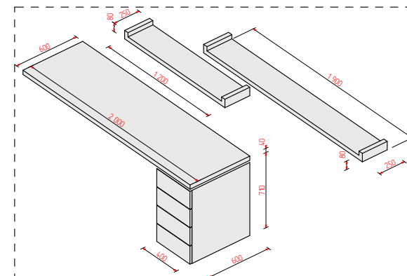
8 Деталь 1:50
