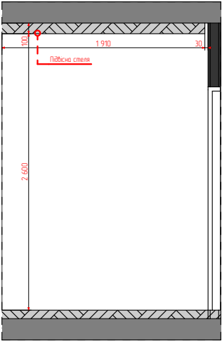
3 Перетин 1:50
