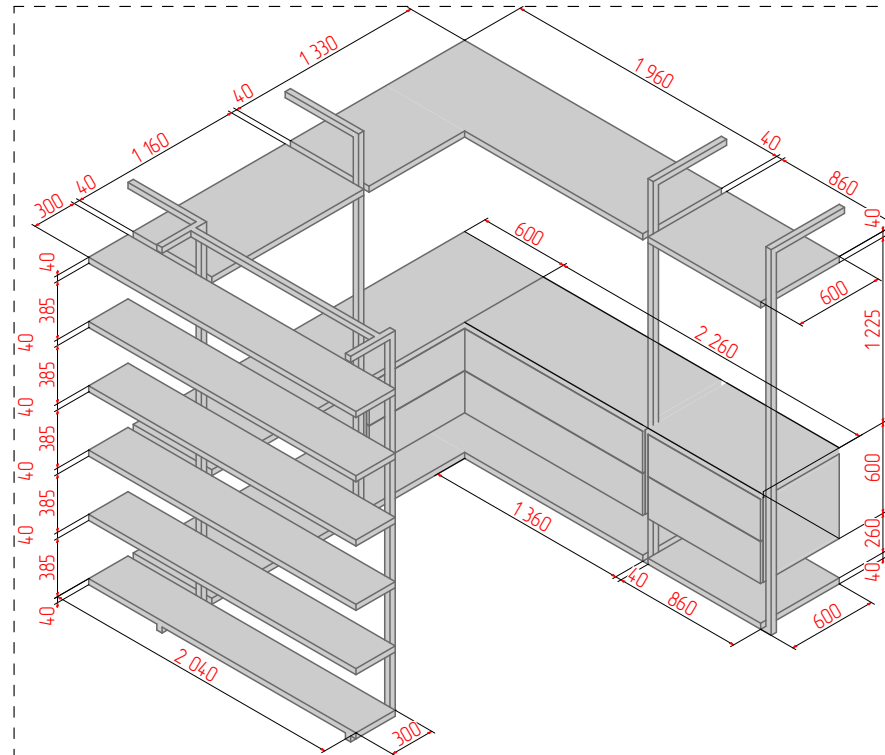
8 Деталь w 1:50
