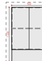
12 Деталь w 1:50
