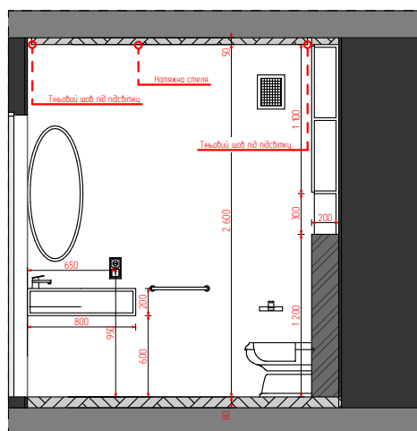
26 Перетин (1) 1:50
