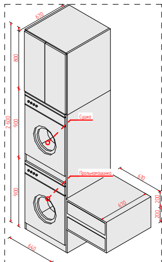
13 Деталь q 1:50
