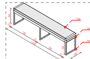
16 Деталь 1:50
