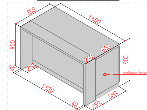
4 Деталь q 1:50
