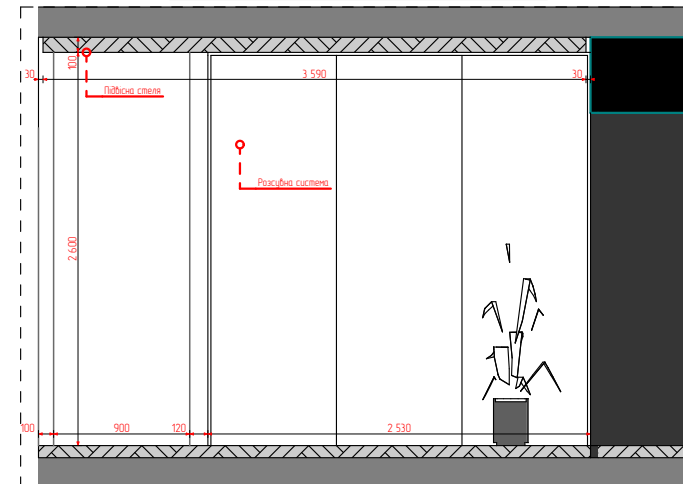
22 Перетин 1:50
