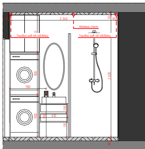
21 Перетин (1) 1:50
