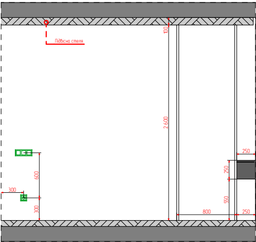
8 Перетин 1:50
