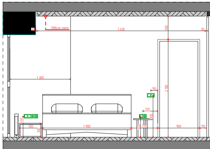
21 Перетин 1:50
