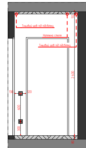
3 Перетин (1) 1:50
