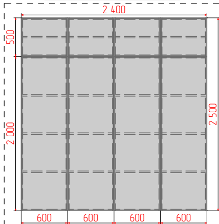
7 Деталь w 1:50
