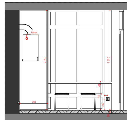
10 Перетин (1) 1:50
