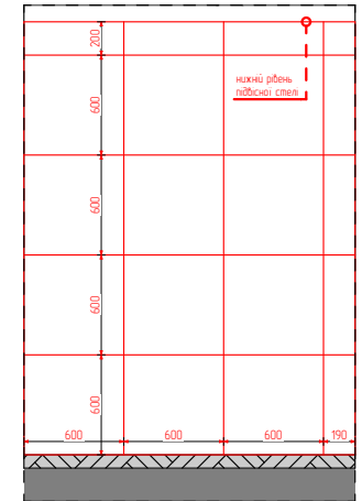
06 Розгортка 1:50
