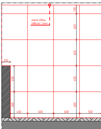
07 Розгортка (1)1:50
