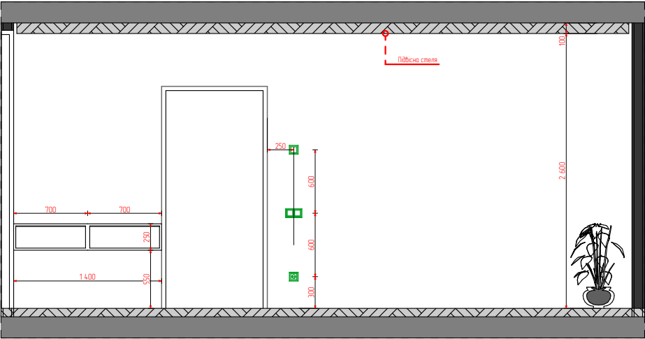
1 Перетин 1:50
