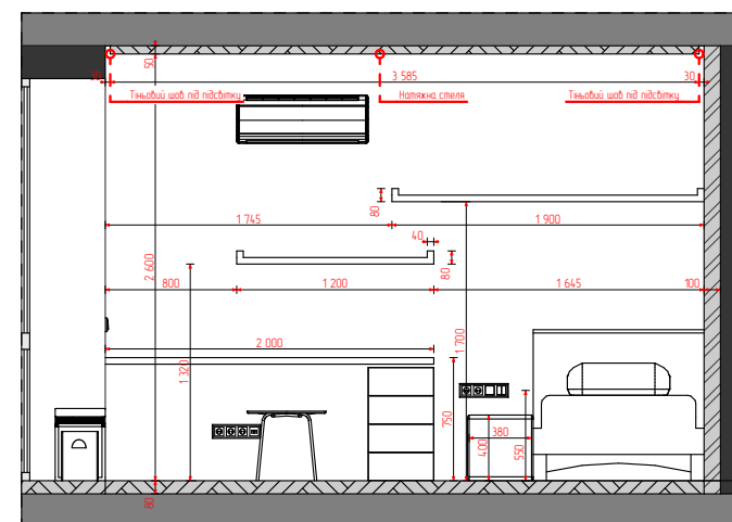
19 Перетин (1) 1:50
