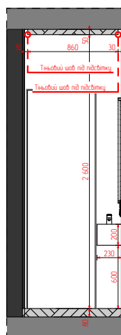
25 Перетин (1) 1:50
