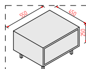
14 Деталь q 1:50
