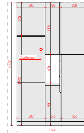
1 Деталь е 1:50
