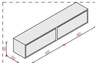
5 Деталь 1:50
