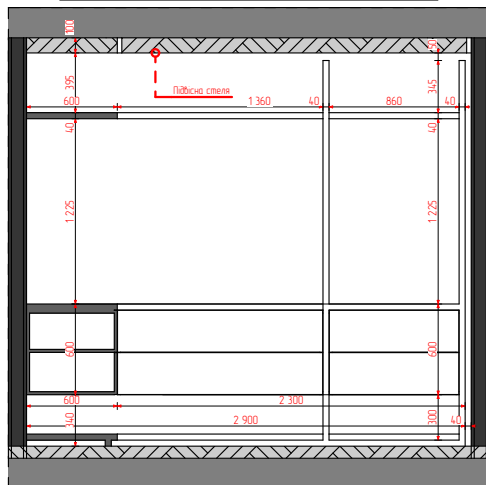
17 Перетин 1:50
