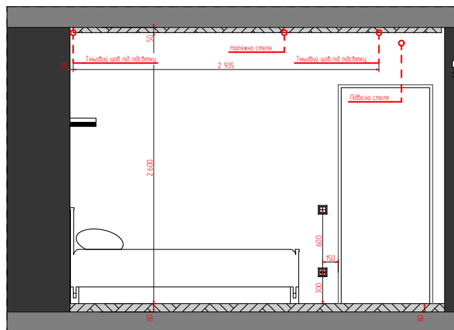
20 Перетин (1) 1:50
