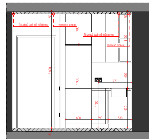
7 Перетин (1) 1:50
