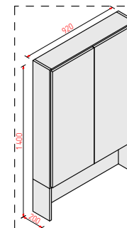
12 Деталь q 1:50
