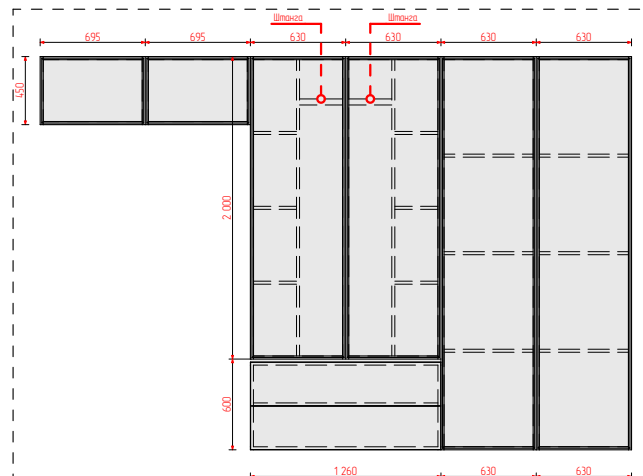
13 Деталь w 1:50
