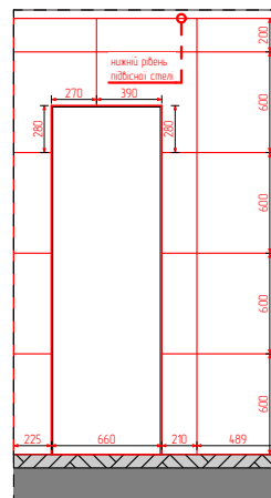
04 Розгортка (1)1:50
