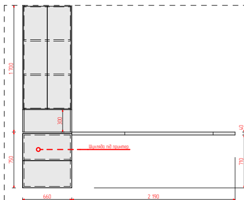
6 Деталь w 1:50
