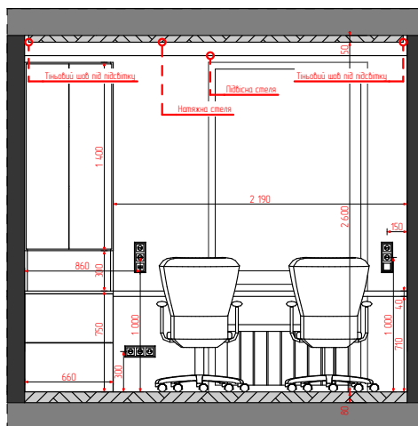
14 Перетин (1) 1:50
