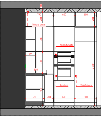
7 Перетин 1:50
