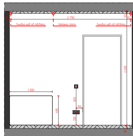
16 Перетин (1) 1:50
